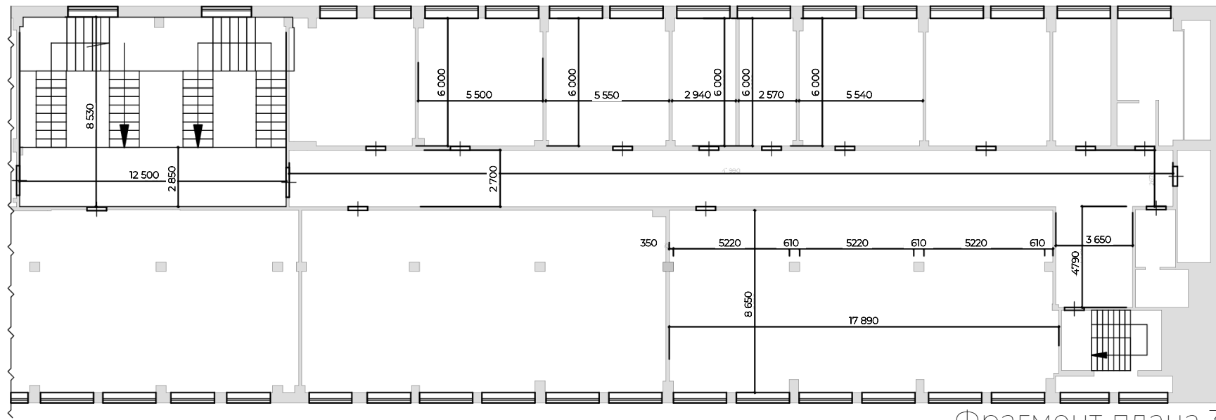
Фрагмент плана 3-го этажа с размерами
